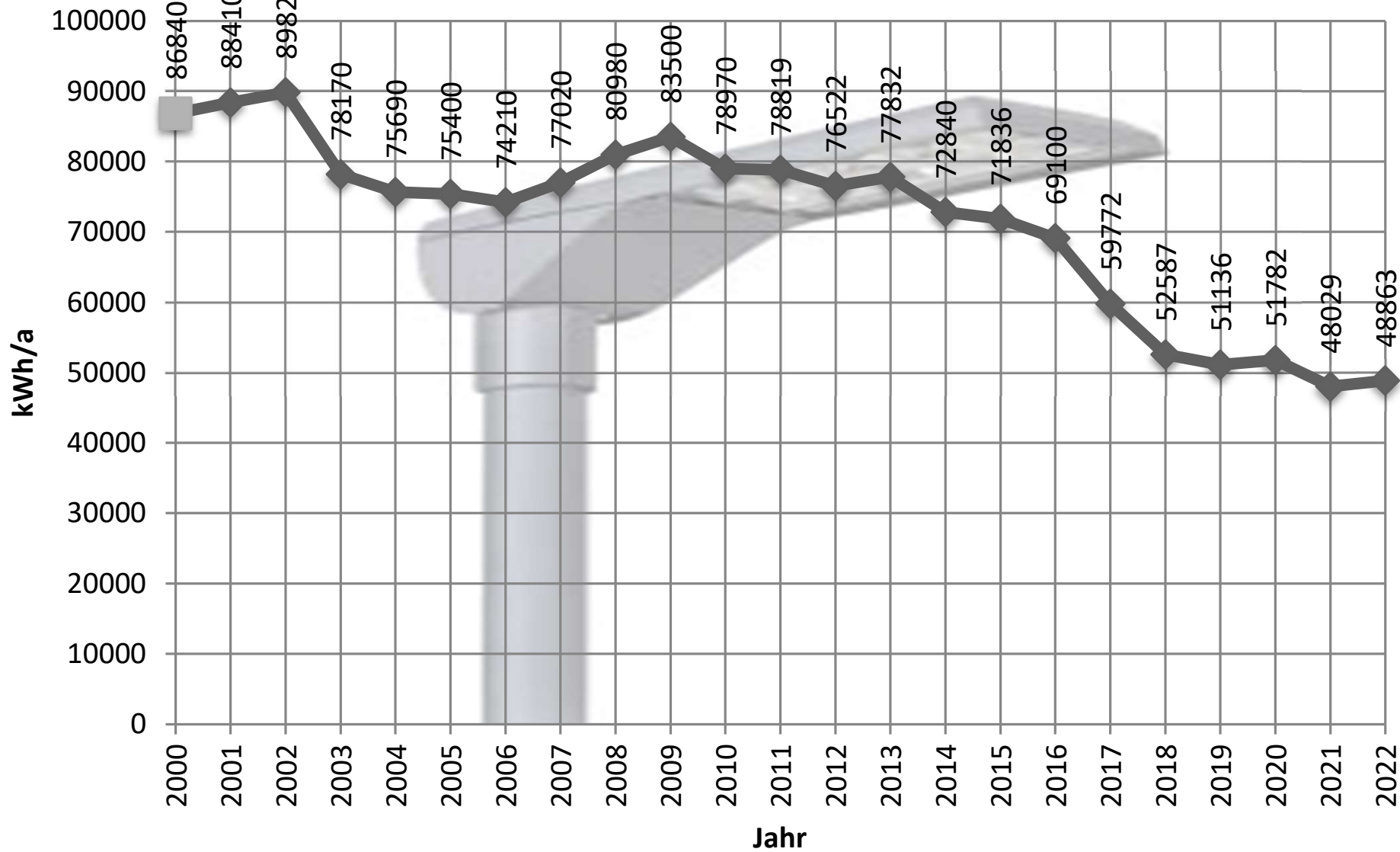
Energie Verbrauch Strassenbeleuchtung in kWh/a, 2000 - 2022 Gem. Barga
